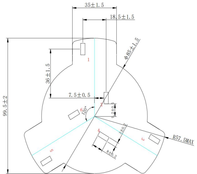
底视图
